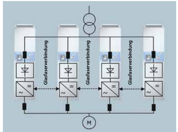
Beispiel einer VACON DriveSynch-Konfiguration.
